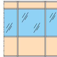
► Vitré sur allège avec imposte Partial-height glazed with apron and overpanel
