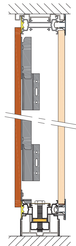
Coupe verticale
