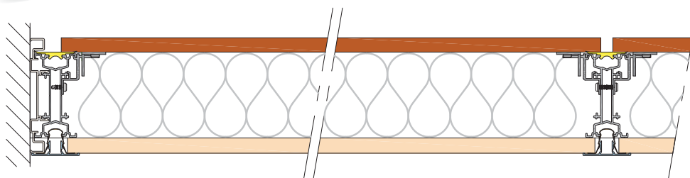
Coupe horizontale
