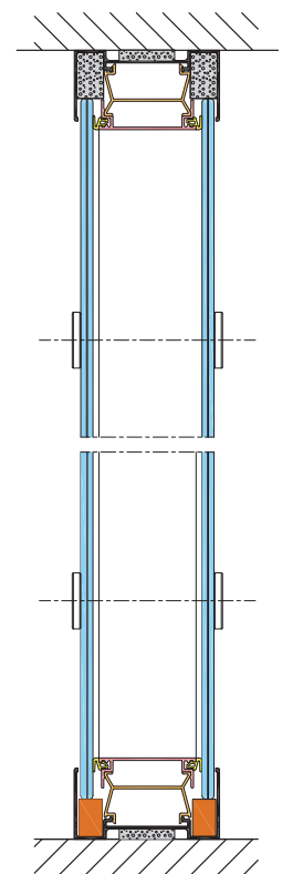
Coupe verticale
